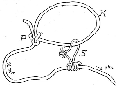
Knotenriss-Sicherung: K Körperschlinge, P Palstek, S Sturzschnge
