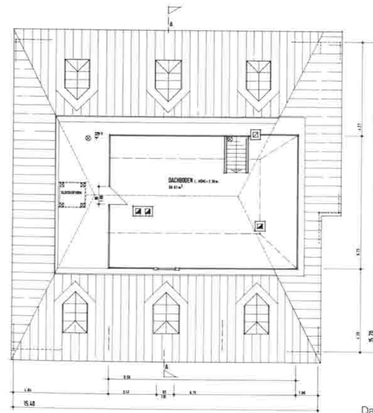
Dachgeschoß
