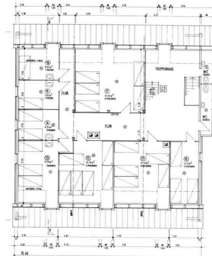
2. Obergeschoß
