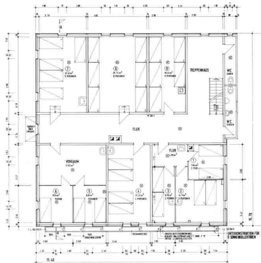
1. Obergeschoß
