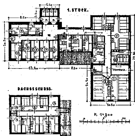
Links das Obergeschoß der Hütte und das Dachgeschoß des Schlafhauses
