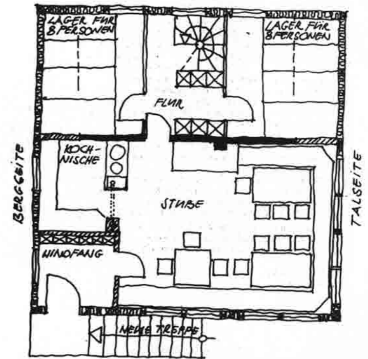
GRUNDRISSE DES OBERGESCHOSSES
