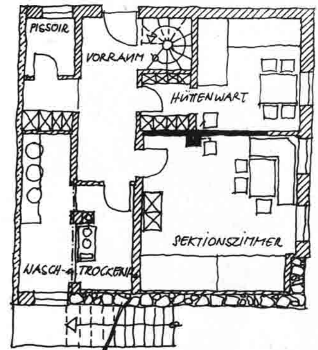
GRUNDRISSE DES UNTERGESCHOSSES
