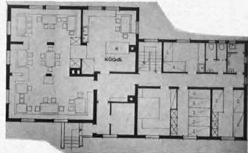
Hamburger Skiheim • Grundriß Erdgeschoß
