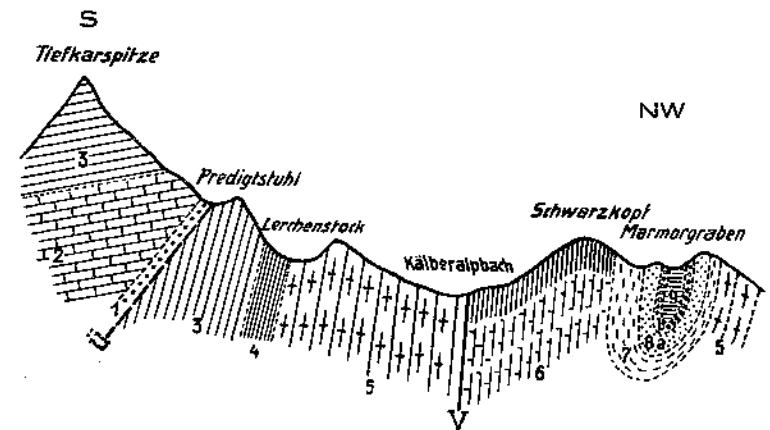
1 Reichenhaller Schichten, 2 Muschelkalk, 3 Wettersteinkalk, 4 Raibler Schichten, 5 Hauptdolomit, 6 Plattenkalk, 7 Rössener Schichten, 8a unterer Jura, 8b oberer Jura, 9 Neokom. U = Überschiebung; V = Verwerfung.
