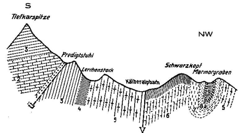
1 Reichenhaller Schichten, 2 Muschelkalk, 3 Wettersteinkalk, 4 Raibler Schichten, 5 Hauptdolomit, 6 Plattenkalk, 7 Kössener Schichten, 8a unterer Jura, 8b oberer Jura, 9 Neokom. U = Überschiebung; V = Verwerfung.
