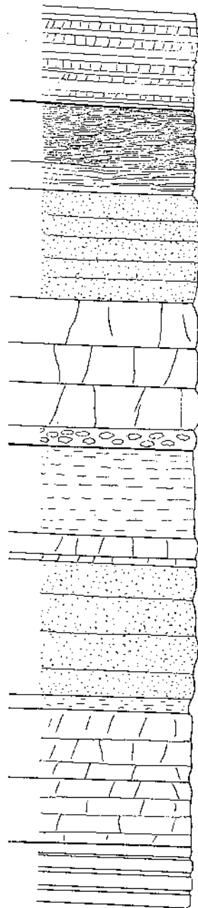
Fig. 2. Profil vom Fonsjoch nach C. Schwager. (1:250 nat. Grösse.)
