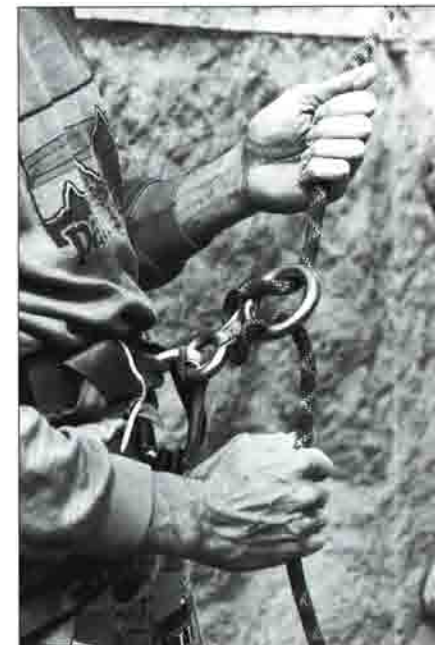
Sicherungstechnik mit Abseilachter
