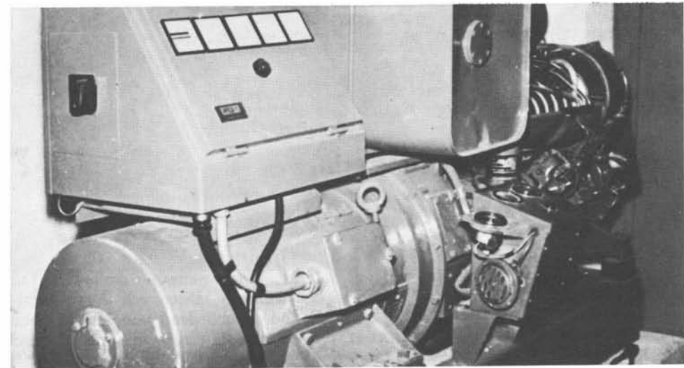
Seilbahn-Diesel-Elektro-Aggregat
