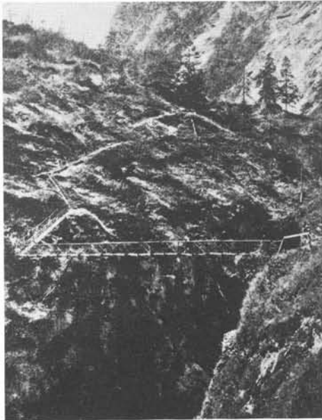
Brücke über die Höllentalklamm im Jahre 1888
