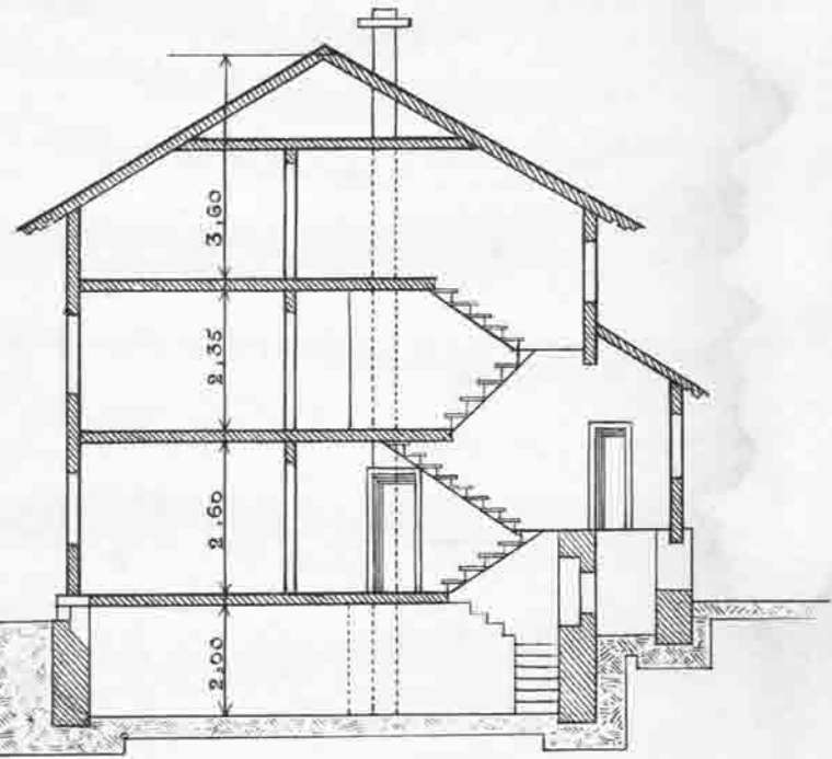
Querschnitt.
