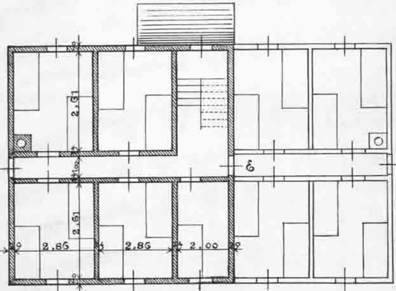
Erster Stock.
