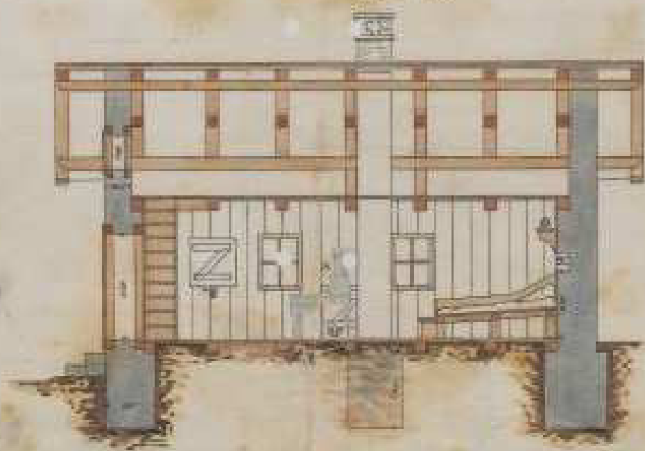
Längenschnitt.
