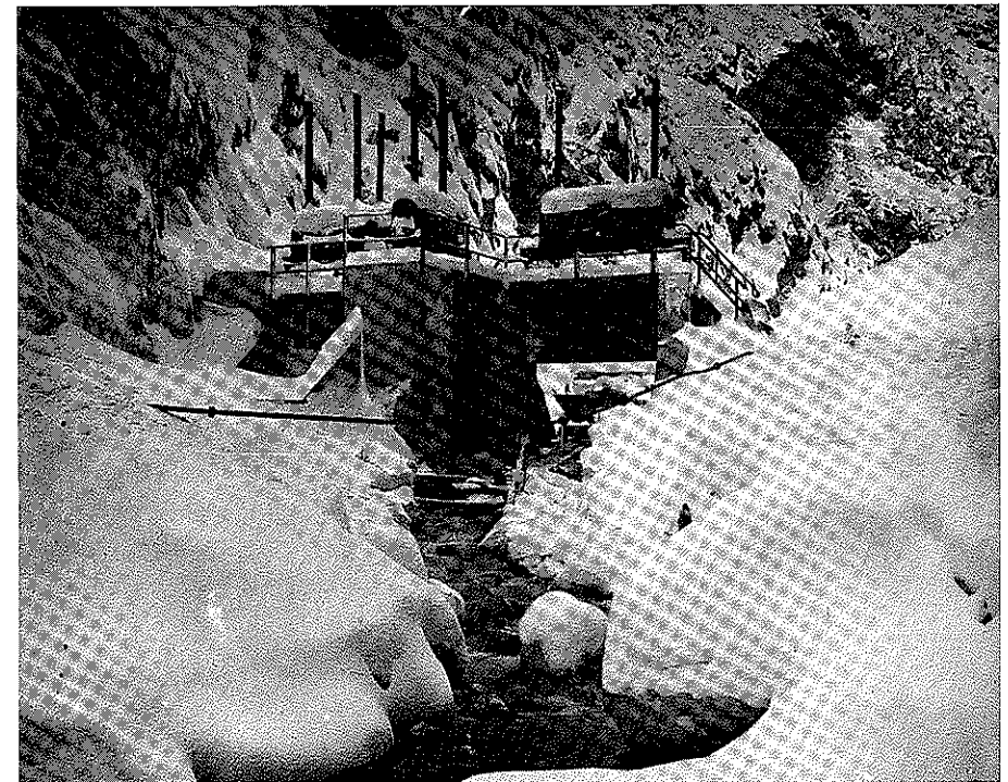
Die Wasserfassung des Hammersbaches kurz nach seiner Fertigstellung im Winter 1916/17, links beginnt der Zuleitungskanal zum Kraftwerk.
