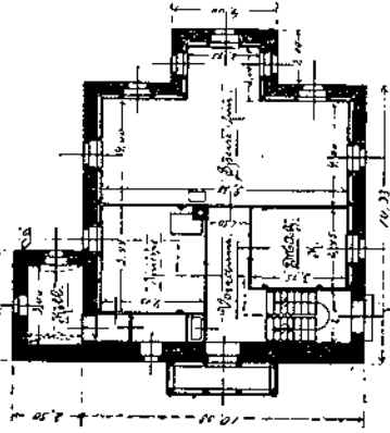
— Untergeschoss —
