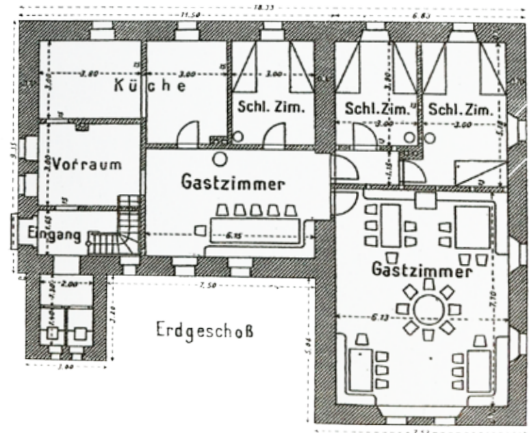
oben: Der Grundriss der Kasseler Hütte in der Rieserferner Gruppe links oben: Die Neue Kasseler Hütte im Zillertal um 1958 links unten: Die Kasseler Hütte (Rieserferner) 1895
