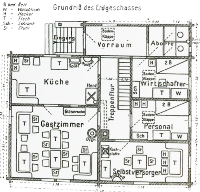
oben: Bauplan der Neuen Kasseler Hütte rechts unten: Die Kasseler Hütte heute
