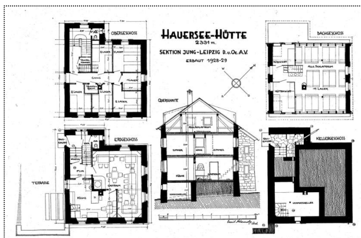
Abb.46: Bauplan der Hauerseehütte. Entwurf: Architekt Adamsky
