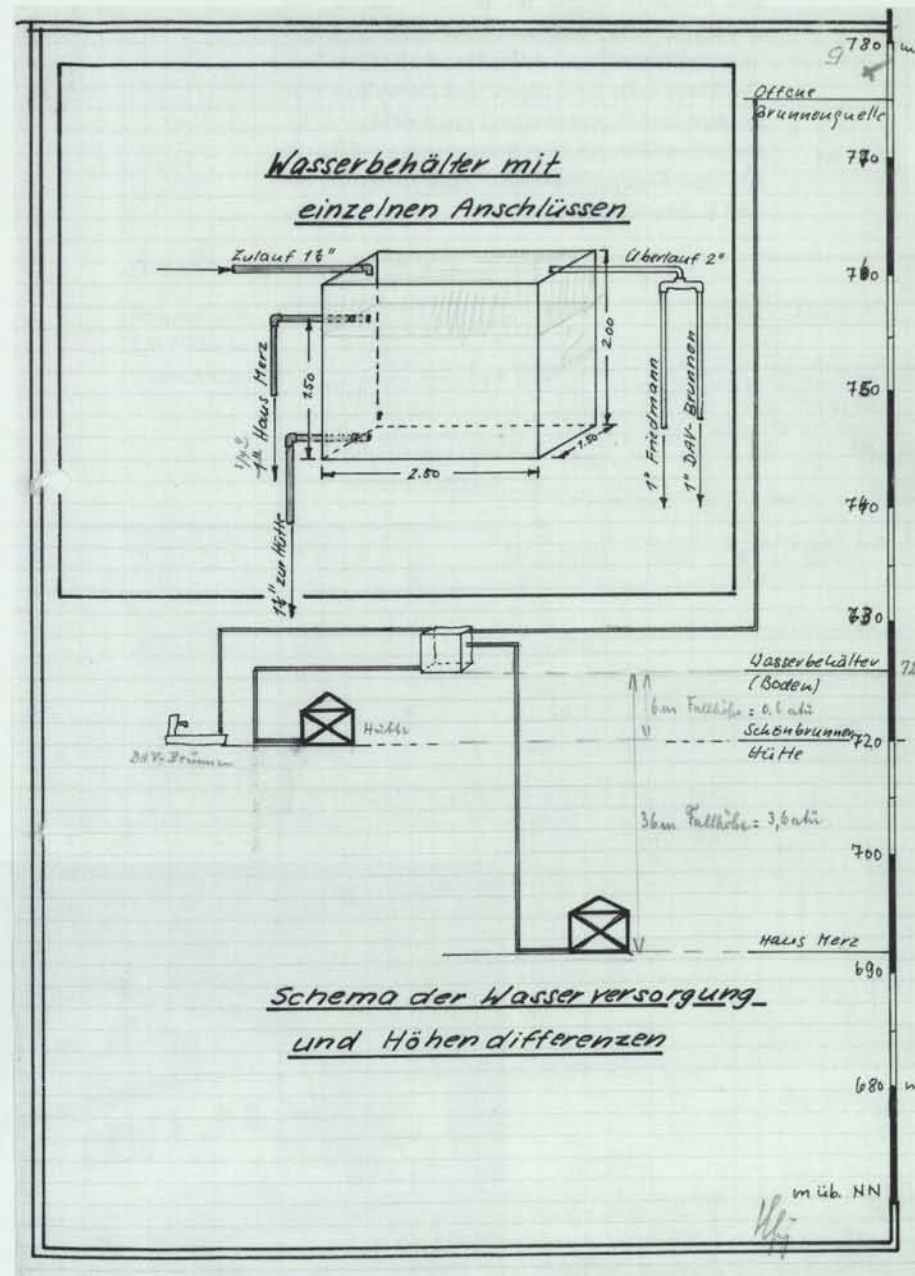
Die Brunnenstube, Auszug aus dem Schema der Wasserversorgung
