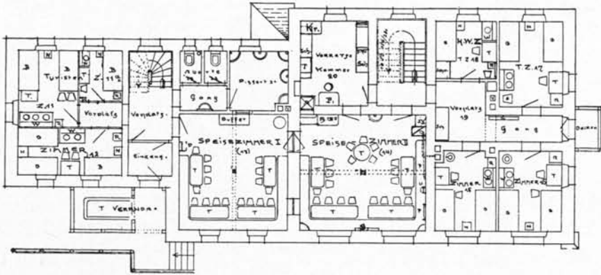
1. Obergeschoß.
