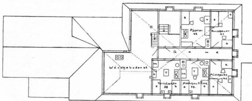
Dachgeschoß.
