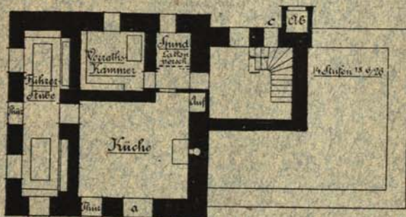
Kellergeschoss.
