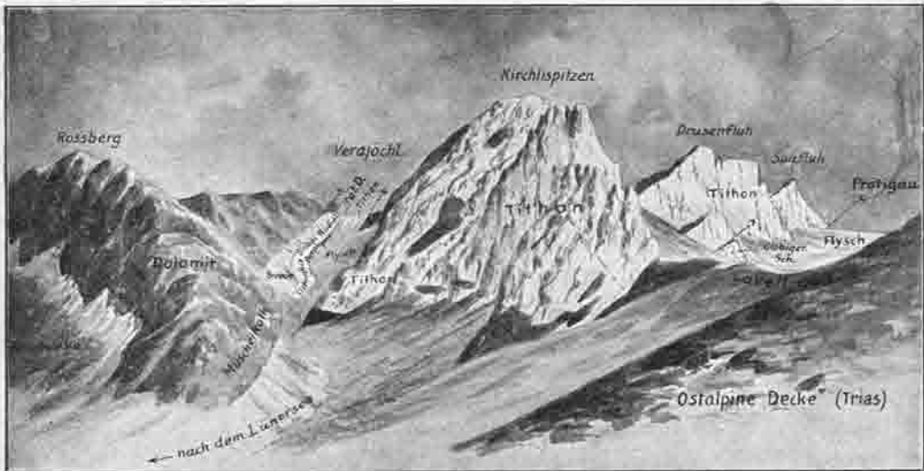
4. Blick vom Cavelljoch auf den Deckenbau des östlichen Raetikons.
