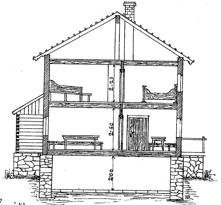
Querschnitt.
