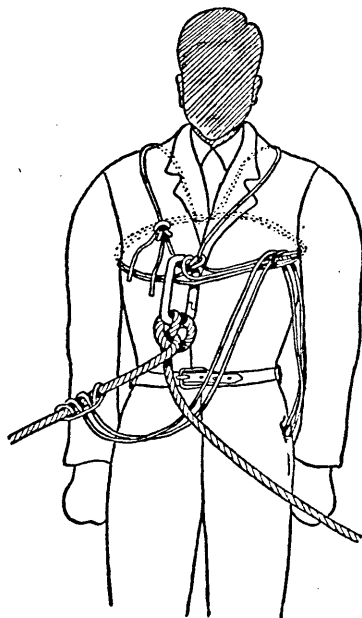
Brustgeschirr für Gletscherfahrten
