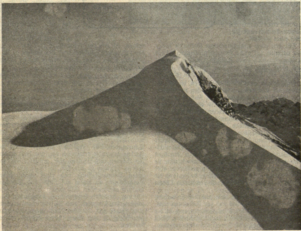
Schneehorn am Hohen Fien (Klein-Walsertal)
