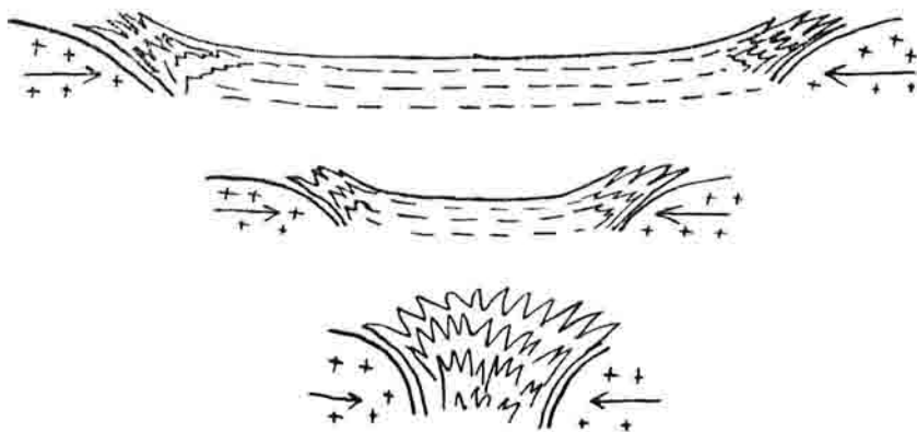
Abb. 1: Auffaltung einer Geosynklinale zwischen zwei Schollenregionen Nach Stille
