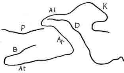
Abb. 5 Das Alpensystem nach Suez 1909
