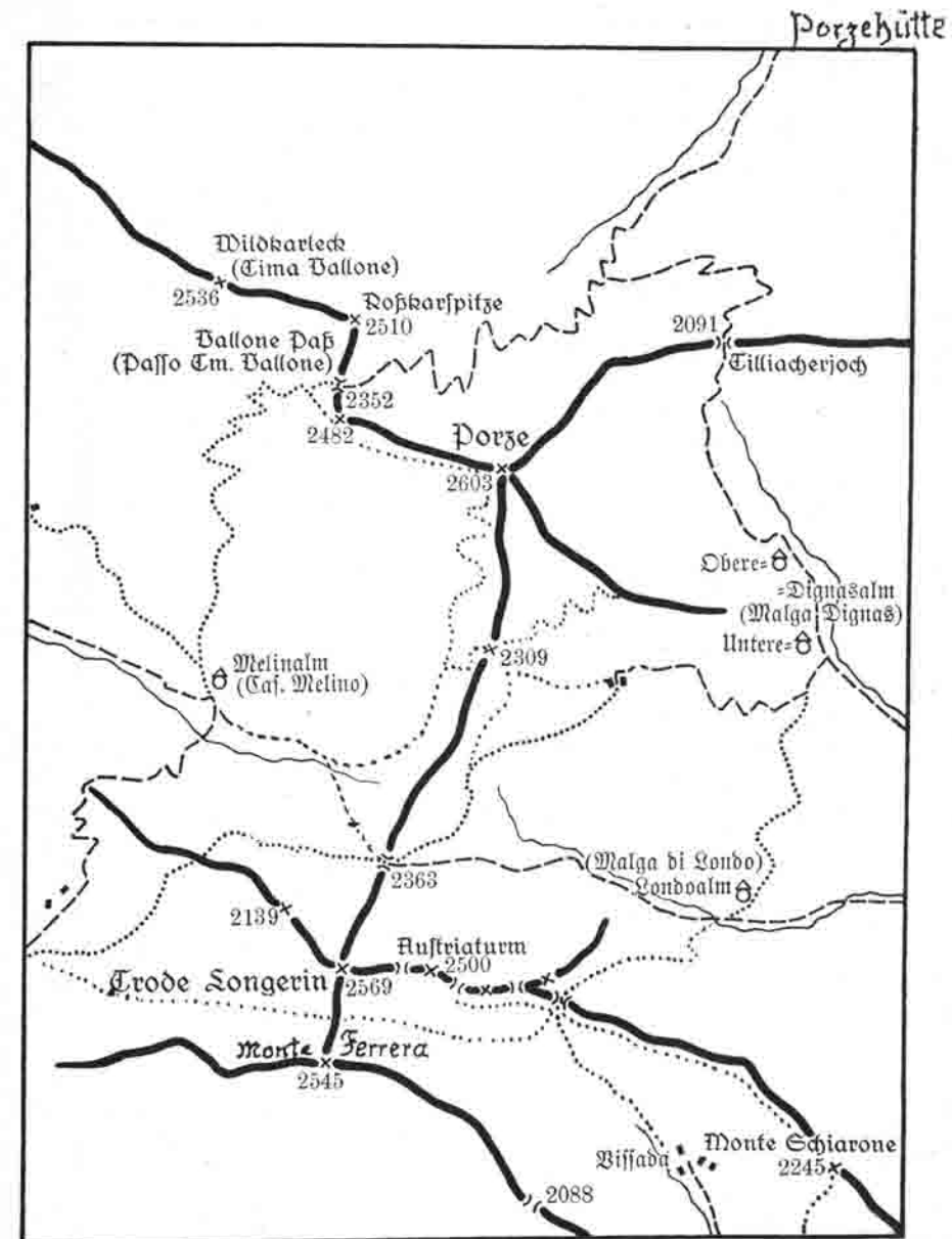
Kammverlaufs-skizze der Crode Longherin-Rete.
