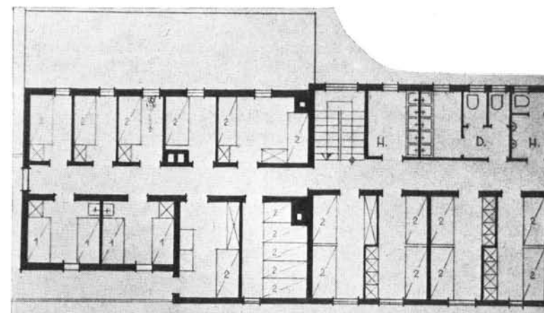
Grundriß Obergeschoß
