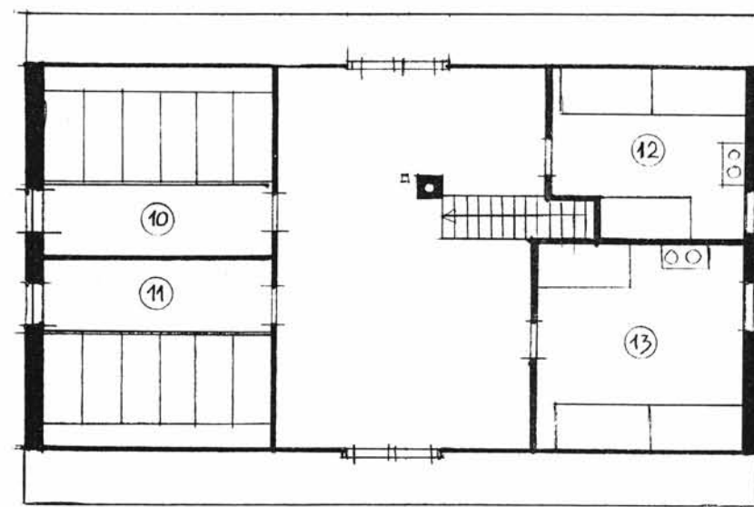
Grundriß Dachgeschoß
