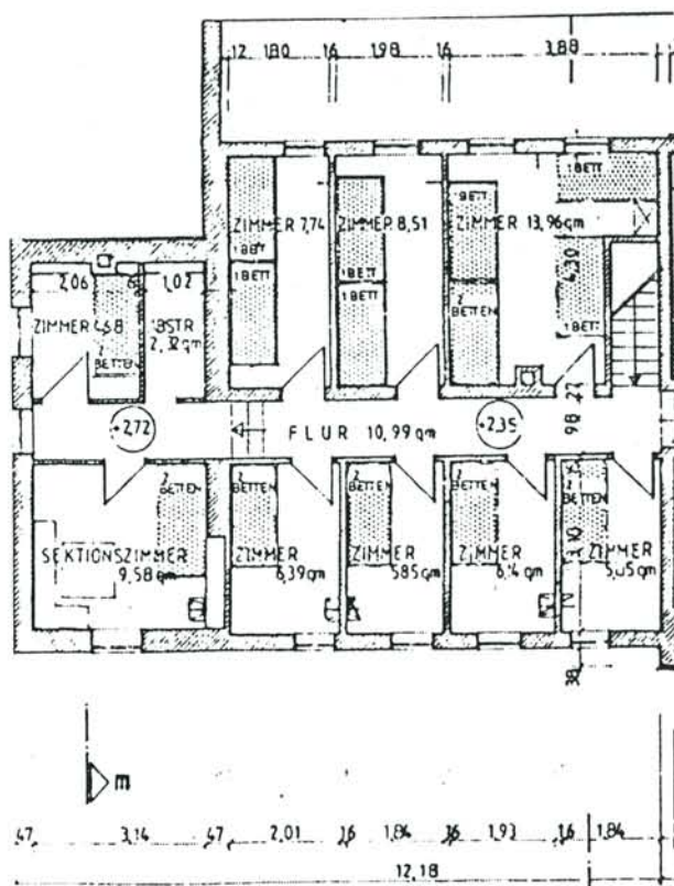
Grundriß Obergeschoß
