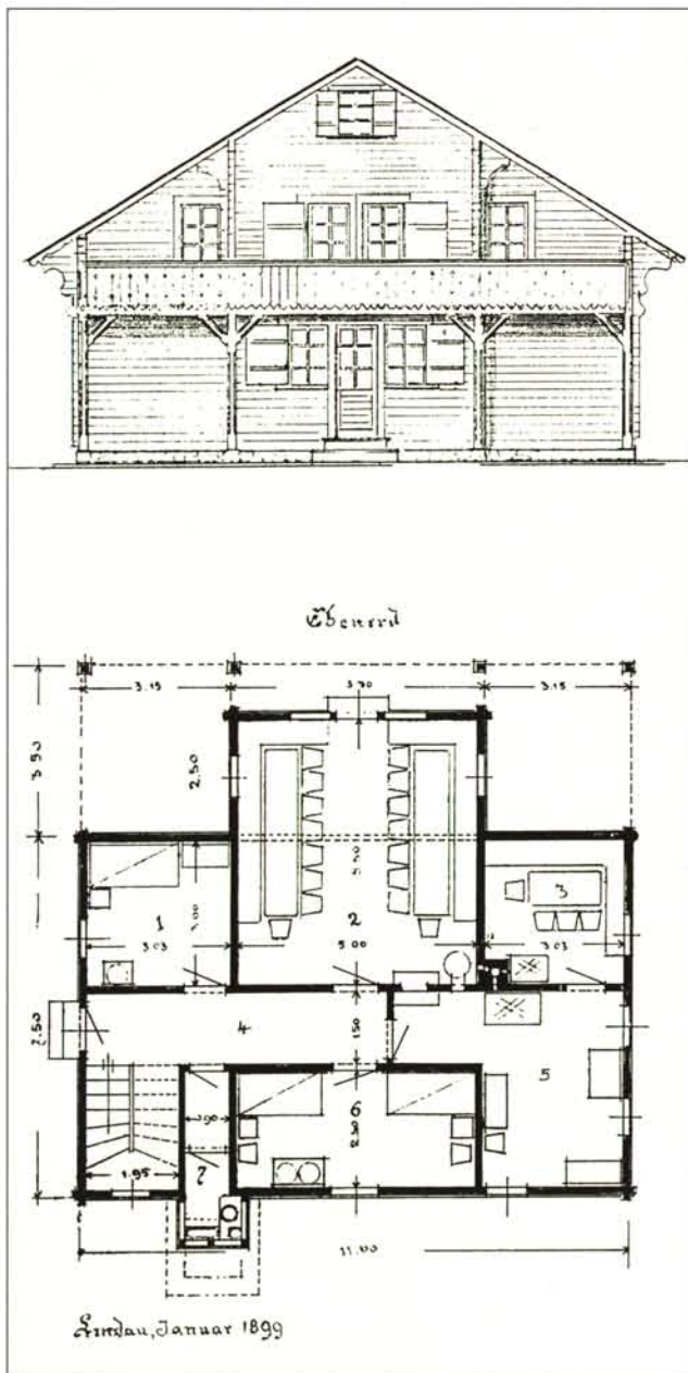
Grundriß und Südostansicht der Lindauer Hütte vom Januar 1899.
