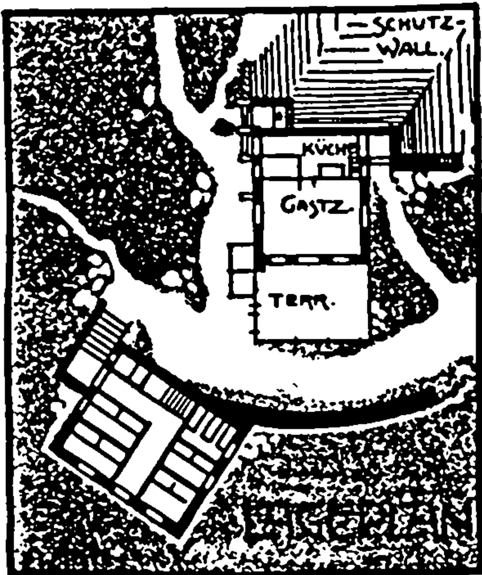
Jetzt bestehende Hütte und die darunter liegende neu projektierte „Mainzer Hütte“, enthält: 9 Zimmer mit 19 Betten, 2 Schlafräume mit 14 Betten, 1 Führerraum mit 10 Betten, Gastzimmer mit Platz für 40 Personen.
