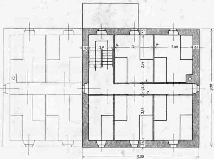
Obergeschoss
