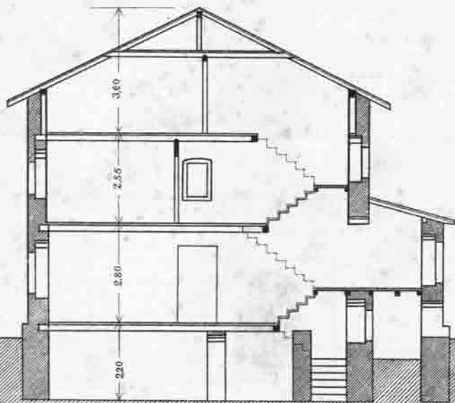
Querschnitt
