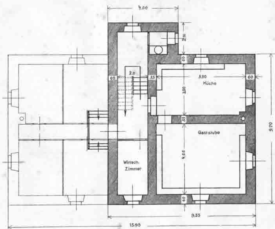
Erdgeschoss
