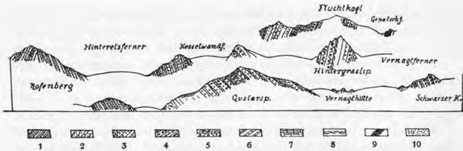
Abb. 5. Geologische Querschnitte durch das Gebiet der Vernagthütte.
