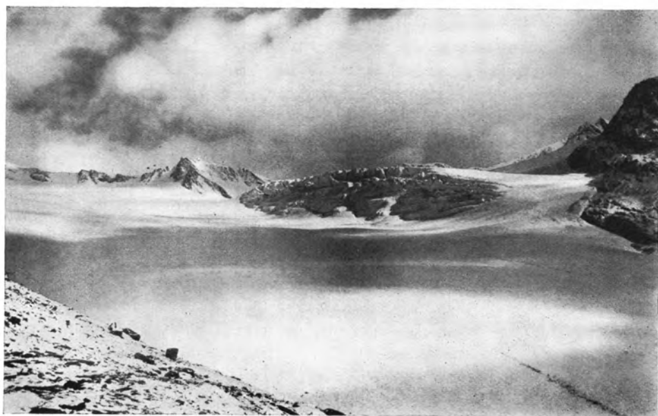
Abb. 10. Großer Eisbruch im Vernagtferner.
