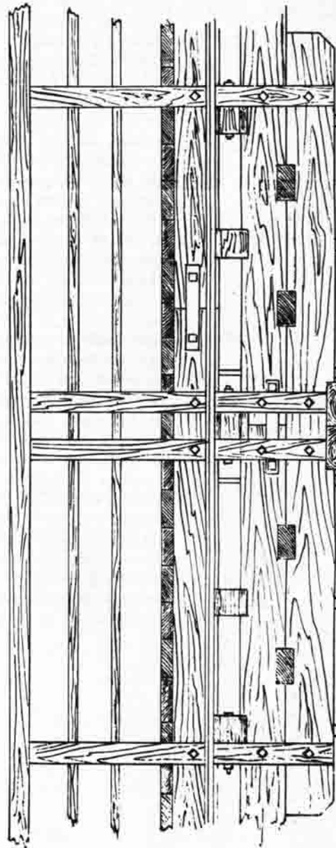
Trägeranflagerung am Mittelgock.
