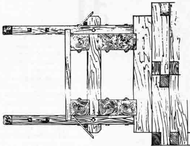
Trägeranflagerung am Mittelgock.
